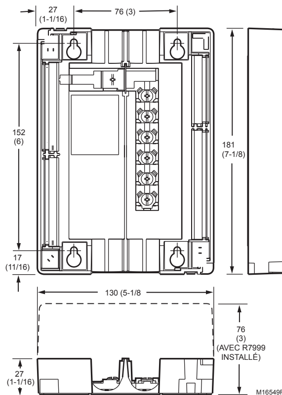
Fig. 1. Encombrement approximatif de la plaque de raccordement universelle ControlLinks mc Q7999A en mm (po).
