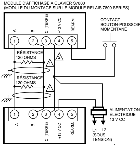
MODULE D’AFFICHAGE A CLAVIER À DISTANCE S7800 ① ②
