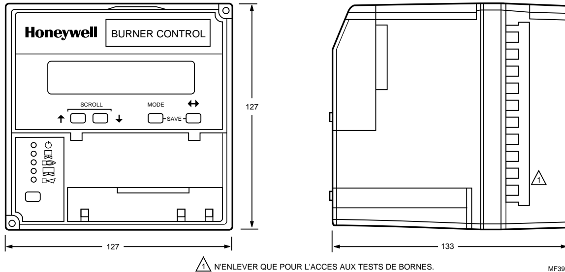
Fig. 1. Encombrement en millimètres du module relais et de l'embase Q7800A.
