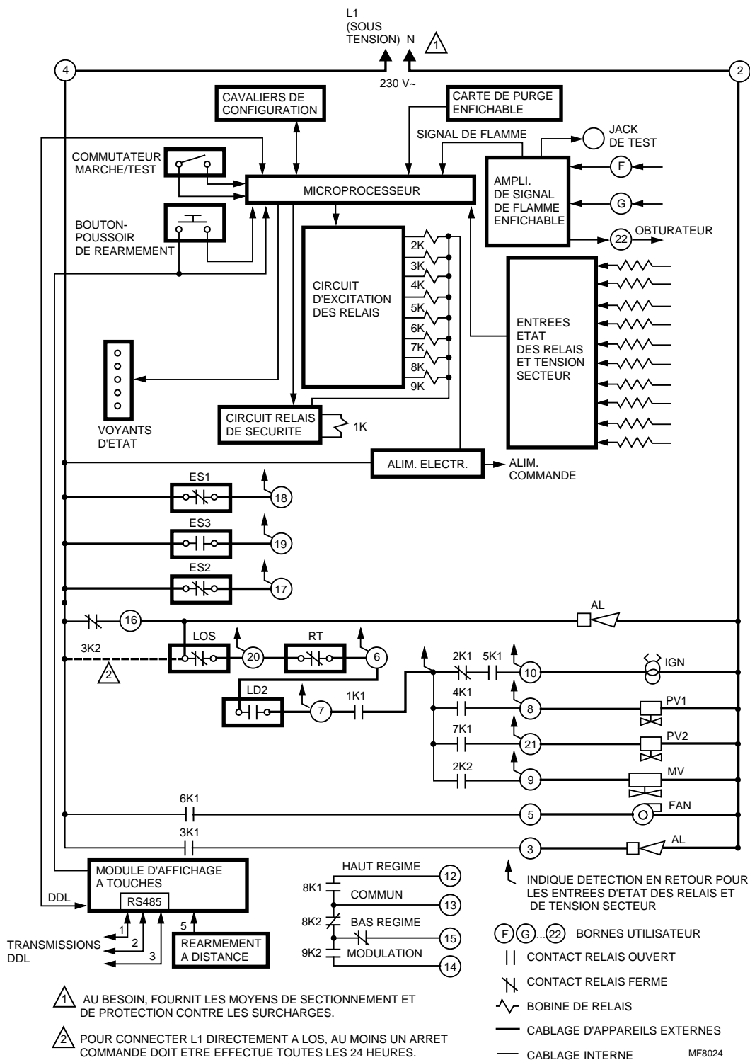
Fig. 3B. Schéma fonctionnel synoptique du module relais EC7850A.
