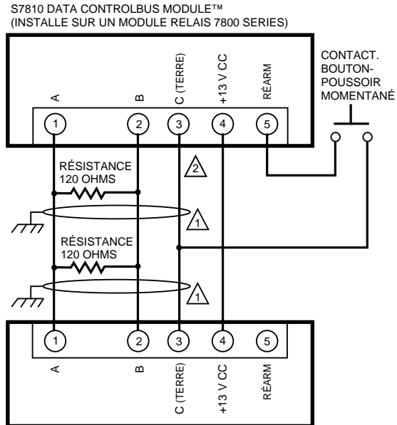
MODULE D’AFFICHAGE A CLAVIER À DISTANCE S7800
