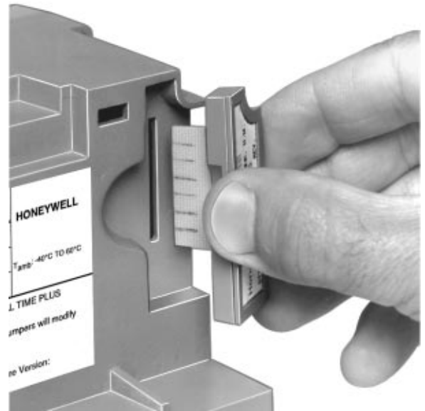
Fig. 8. Installation de la carte de purge ST7800.
