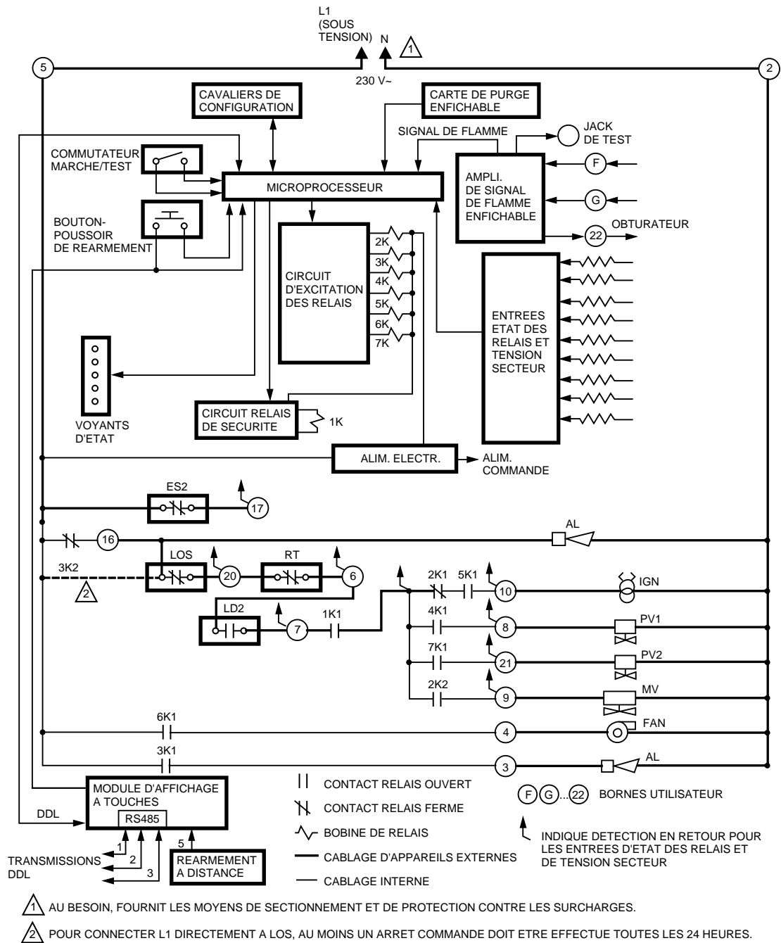
Fig. 3A. Schéma fonctionnel synoptique du module relais EC7830A.
