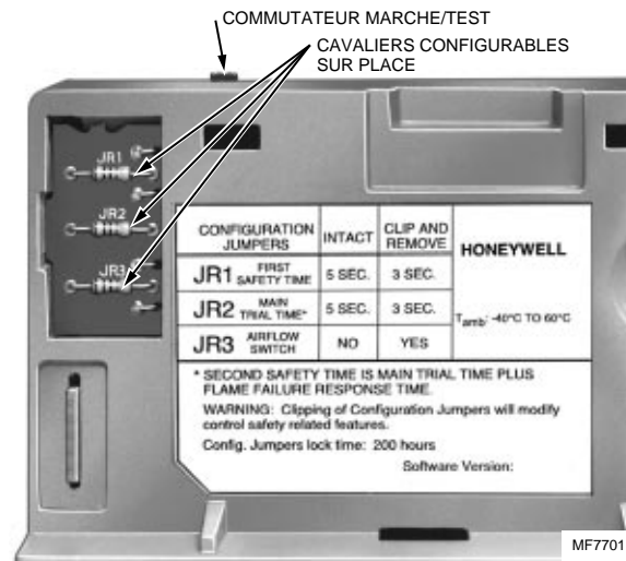
Fig. 15. Cavaliers configurables sur place.
