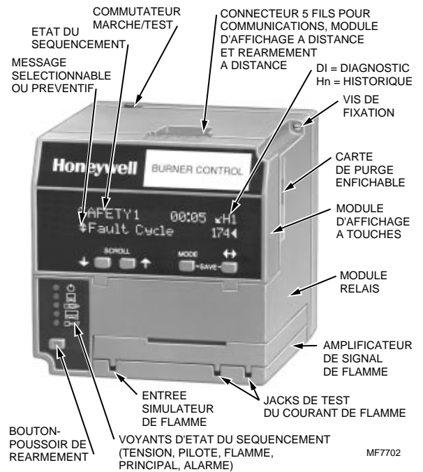
Fig. 17. Module d'affichage à touches et voyants d'état du séquençement (Tableau 5).
