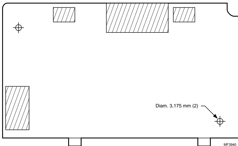
Fig. 23. Montage affleurant d'un gabarit de module d'affichage à touches.
