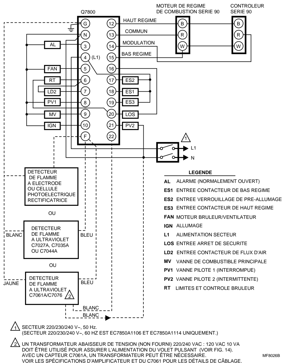
Fig. 4B. Câblage du module relais EC7850A.
