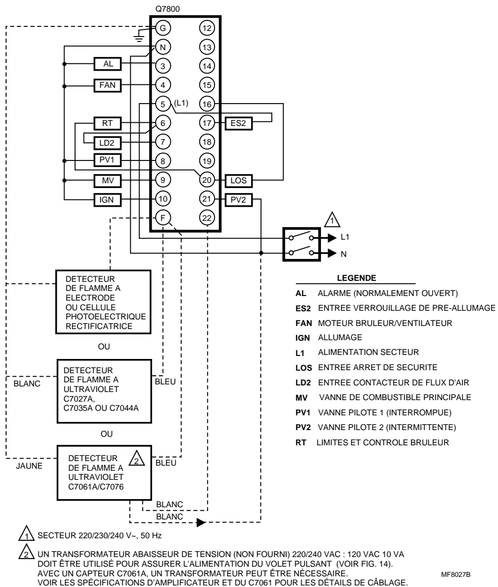
Fig. 4A. Câblage du module relais EC7830A.
