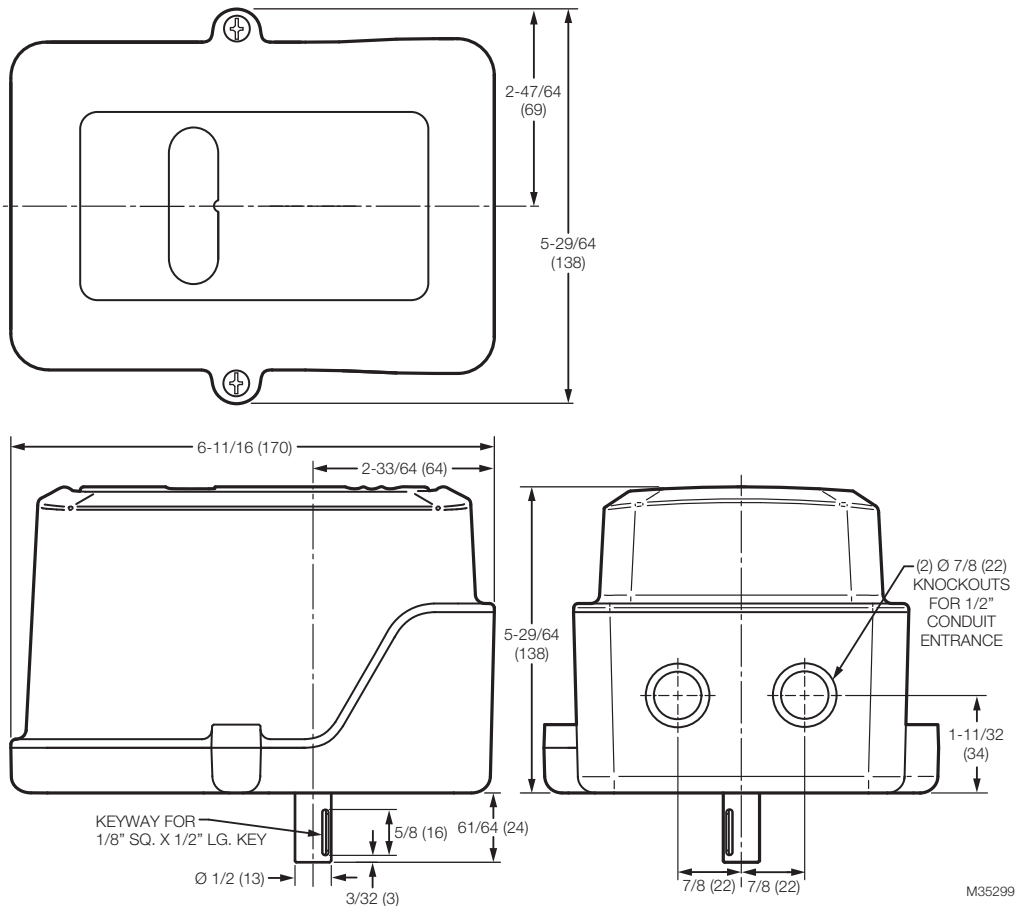
Fig. 1. Dimensiones en mm (in).
